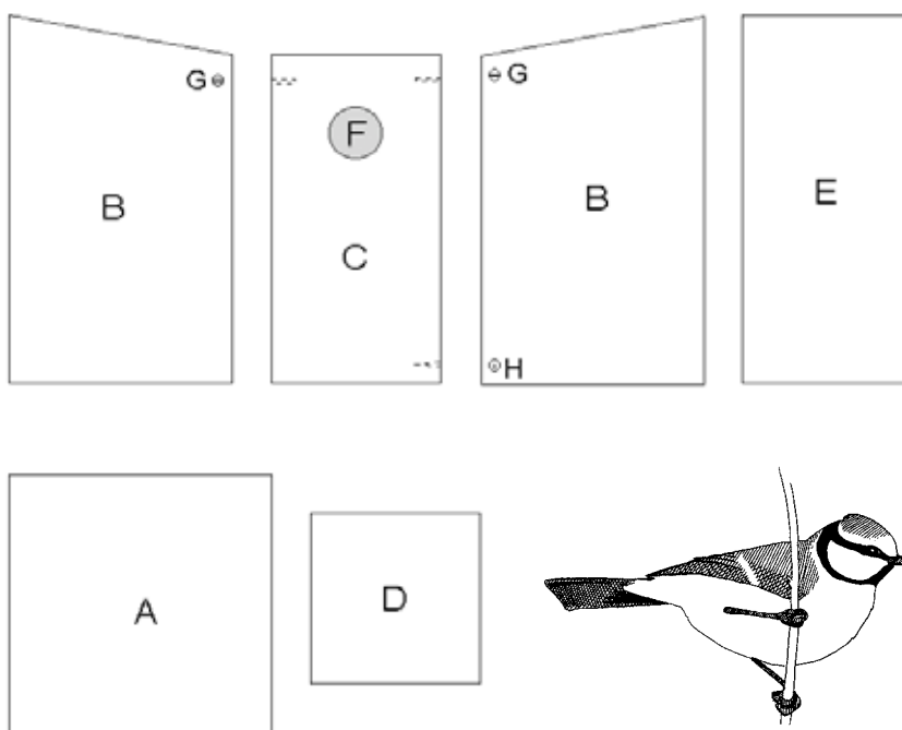
Dimensions pour le nichoir du modèle 1 (données en cm, épaisseur du bois 2 cm):
